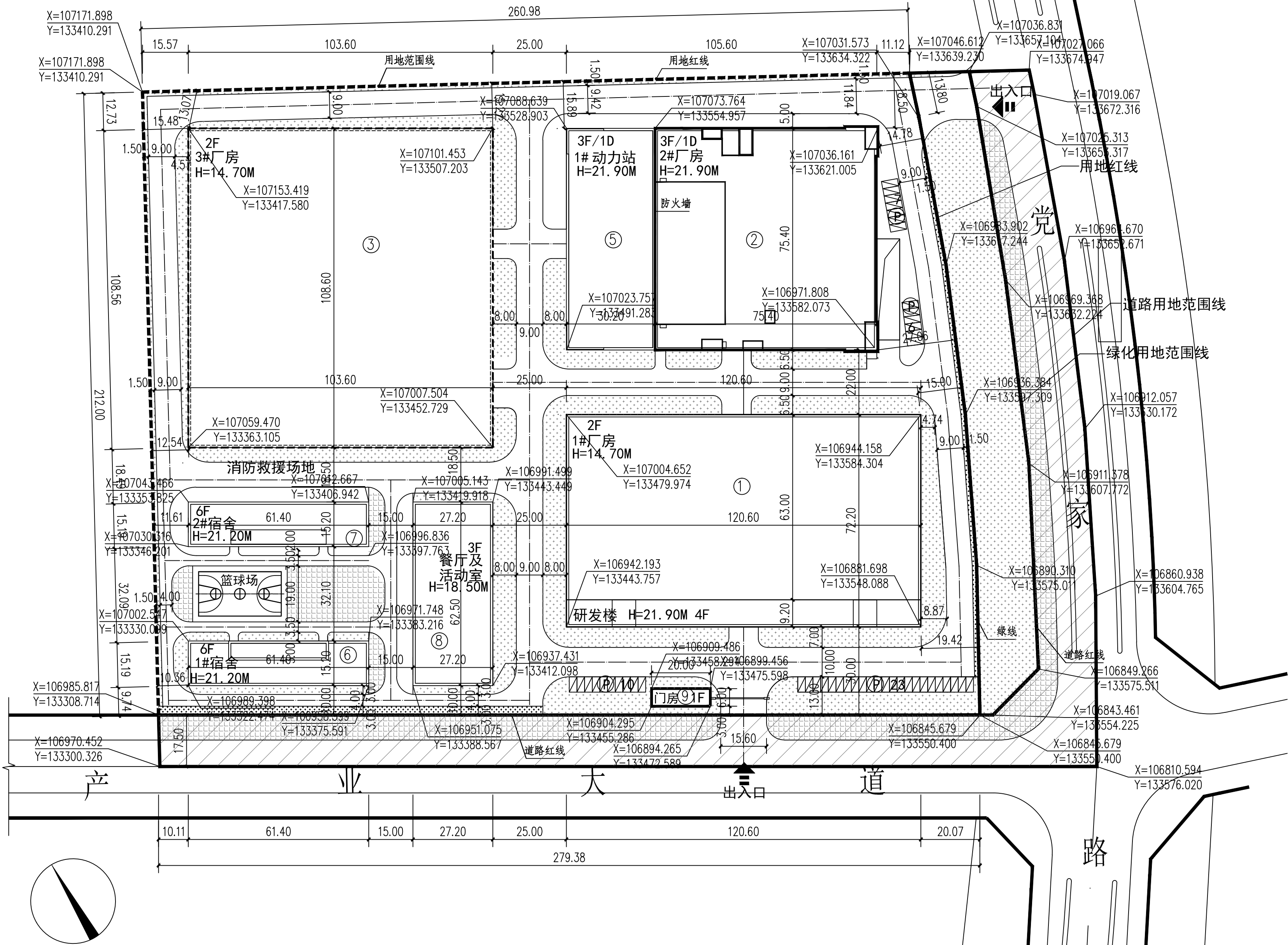
总平面图 1:1000
