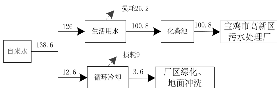
图 2-1 项目水平衡图 (m³/a)
