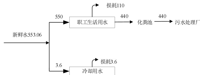
图 2-1 项目水平衡图 单位: \text{m}^3/\text{a}
