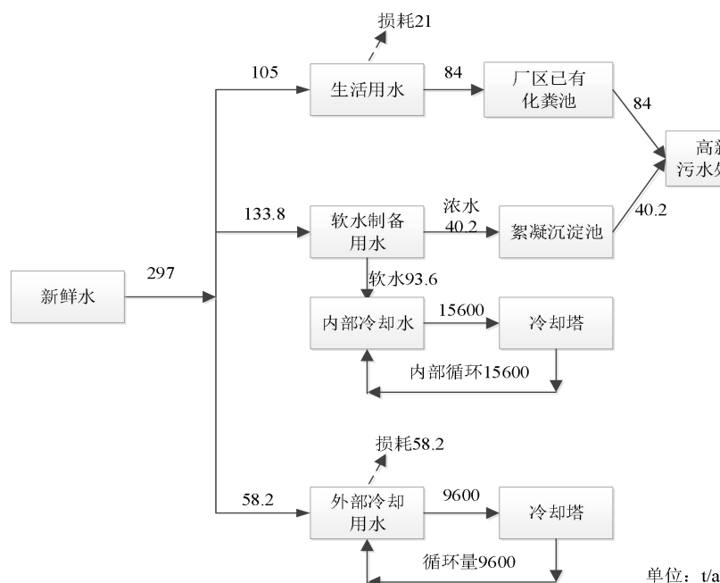
图 3 本项目水平衡图
