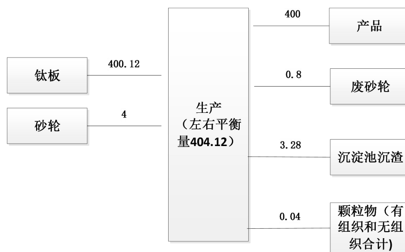
图 2-2 项目物料平衡图
