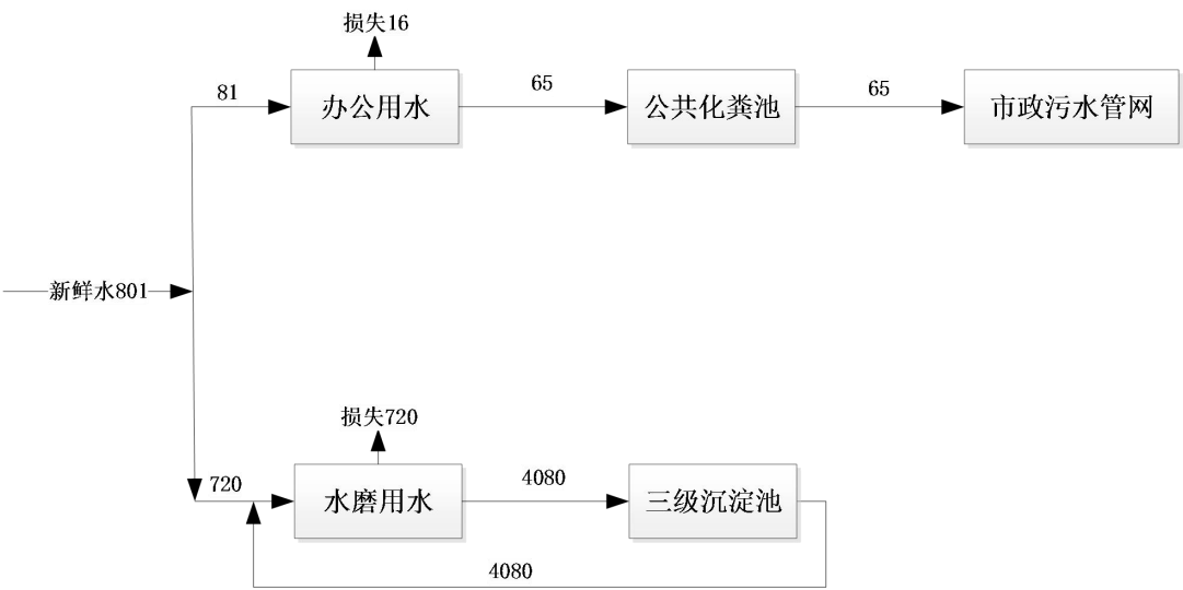
图 2-3 水平衡图 单位：t/a
