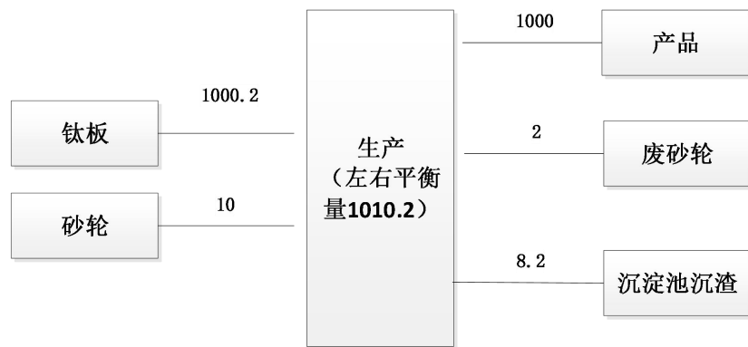
图 2-2 物料平衡图(单位:t/a)
