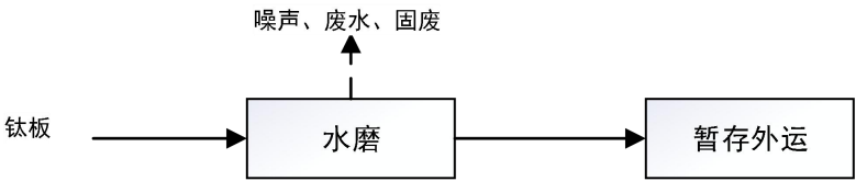
图 2-3 项目钛方、钛棒加工工艺流程及产排污环节图
