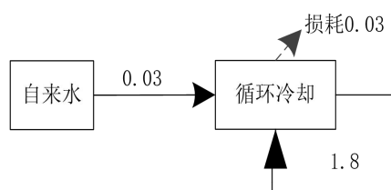
图 2-1 项目水平衡图（m 3 /d）
