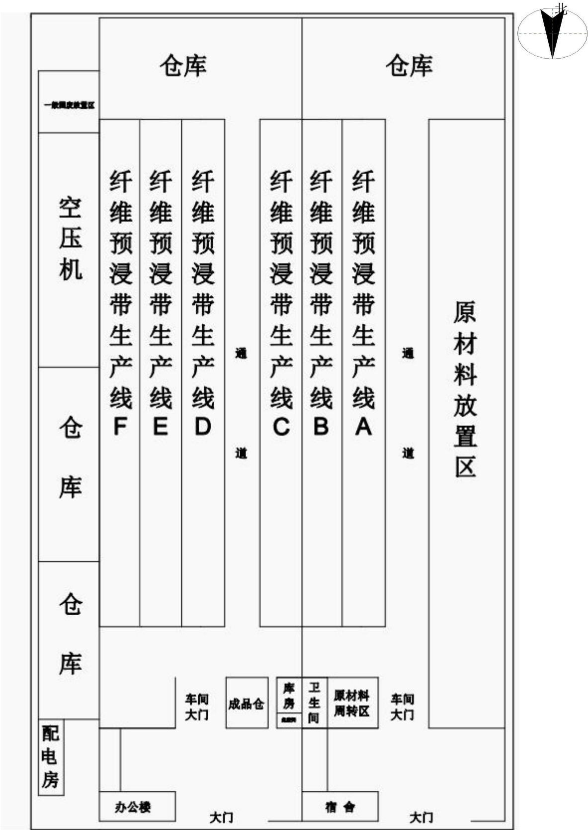
附图 3 建设项目平面布置图（比例尺 1:500）
