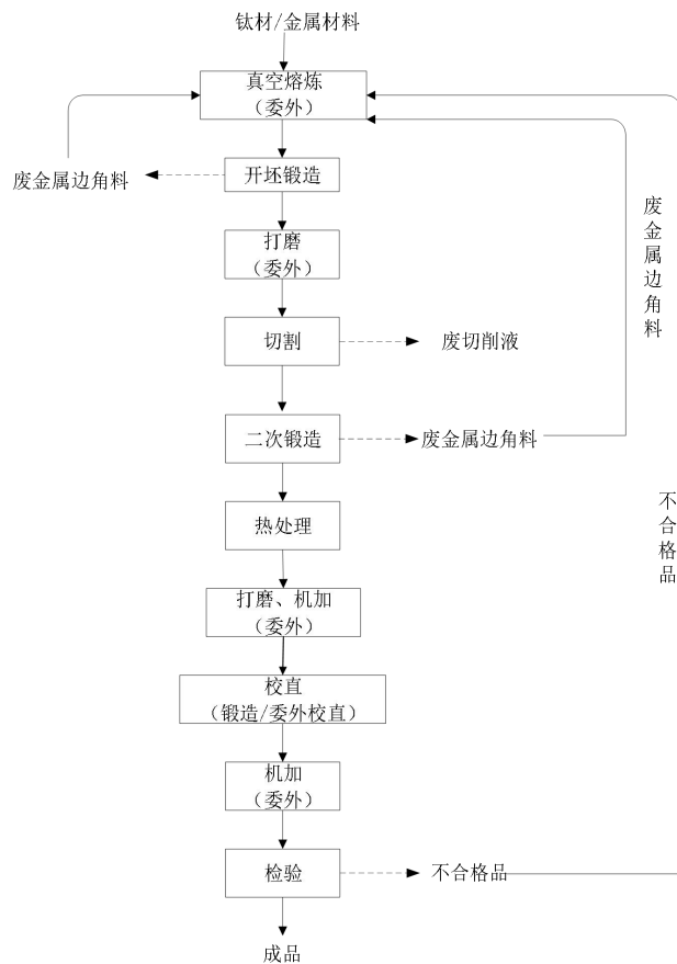
图 2-3 生产工艺流程图
