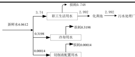
图 2-1 项目水平衡图 单位: \text{m}^3/\text{d}
