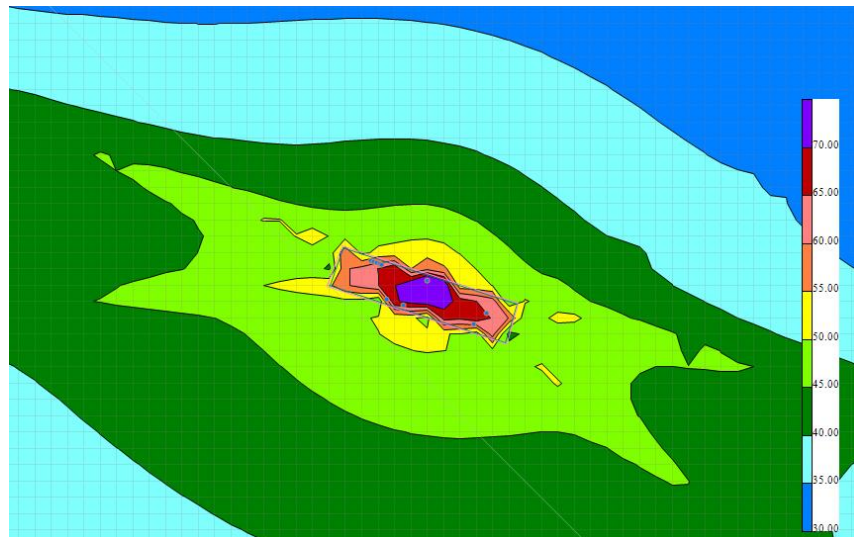
图 4.2 噪声预测等值线图
