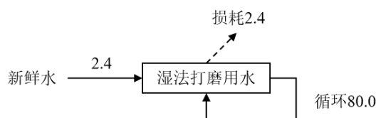
图 2-1 水平衡图 单位: \text{m}^3/\text{d}
