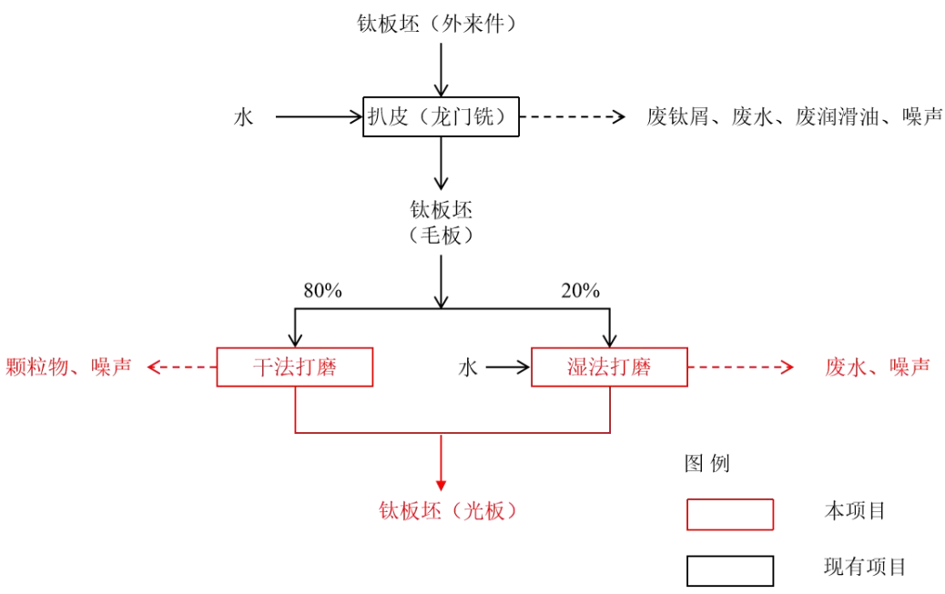
图 2-2 运营期工艺流程及产排污环节示意图
