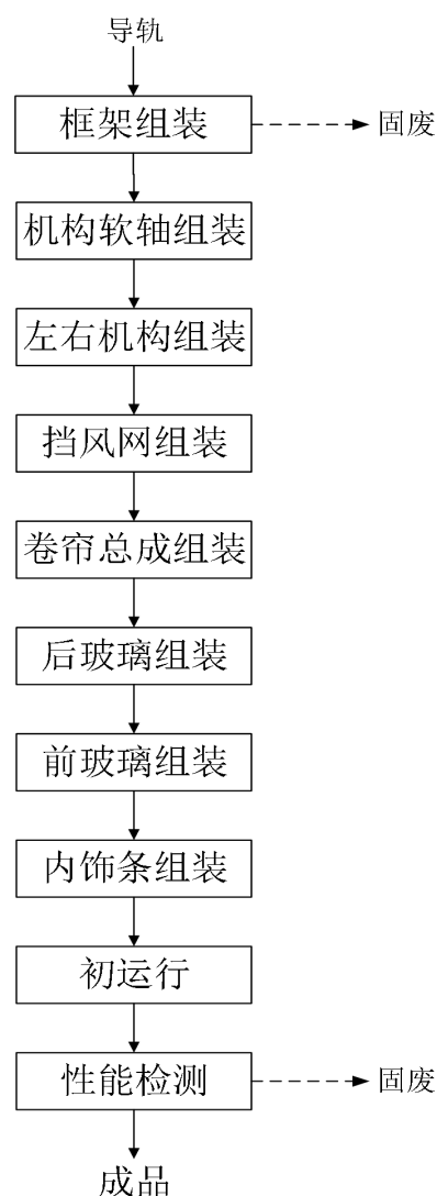
图 2-3 总装生产线工艺流程及产污环节图
