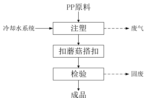
图 2-4 塑料配件生产线工艺流程及产污环节图 工艺流程说明：
