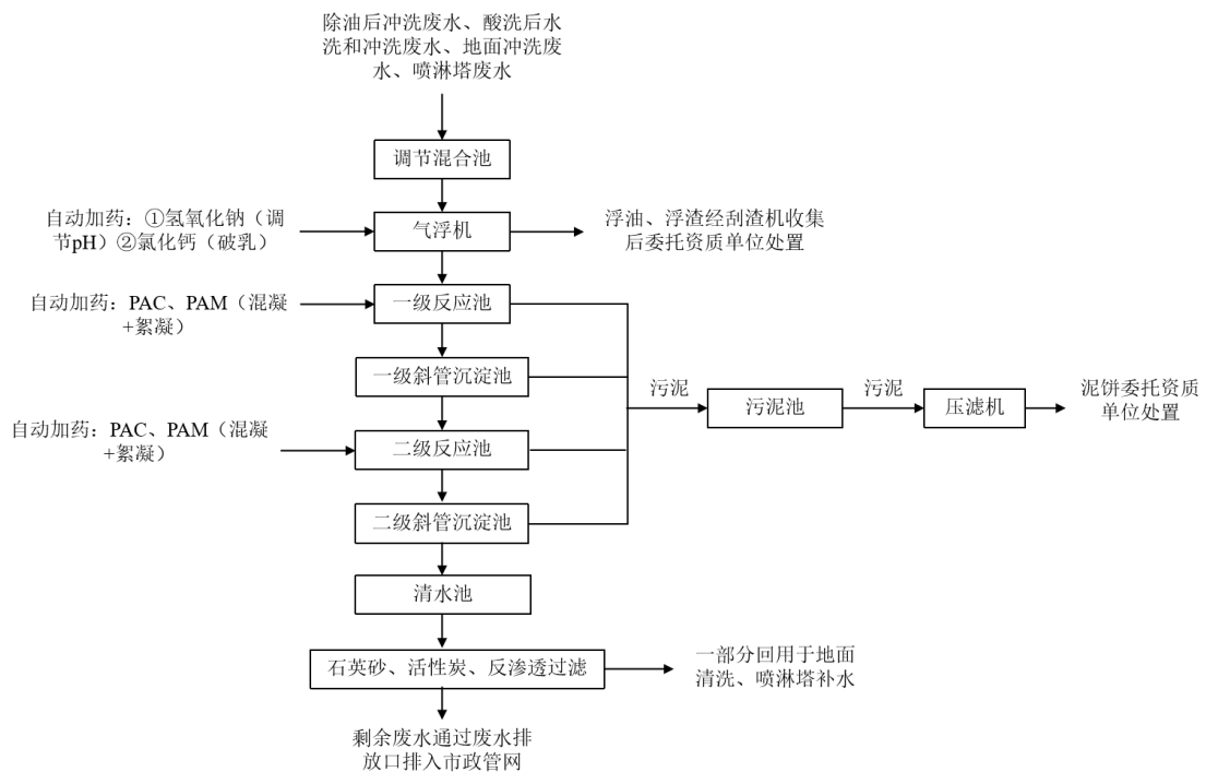
图 4-1 除油酸洗混合废水处理工艺流程图
