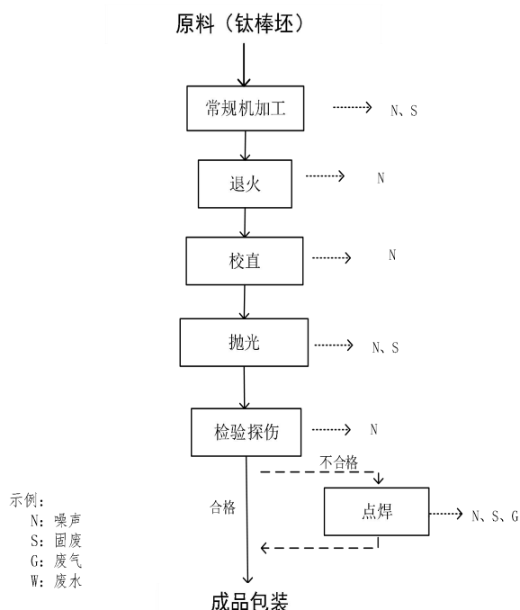
图 2-3 工艺流程及产污环节示意图
