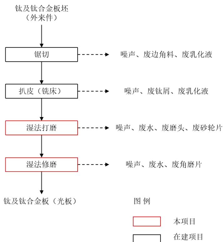
图 2-2 本项目运营期生产工艺流程及产排污环节示意图
