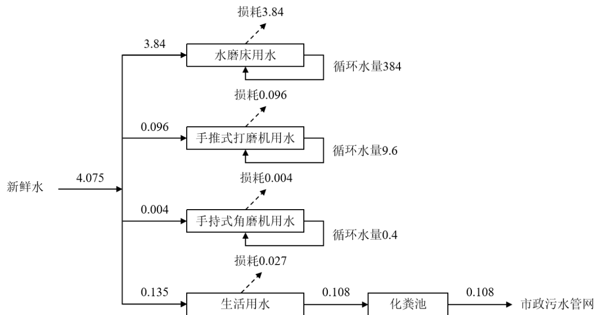
图 2-1 水平衡图 单位: m³/d
