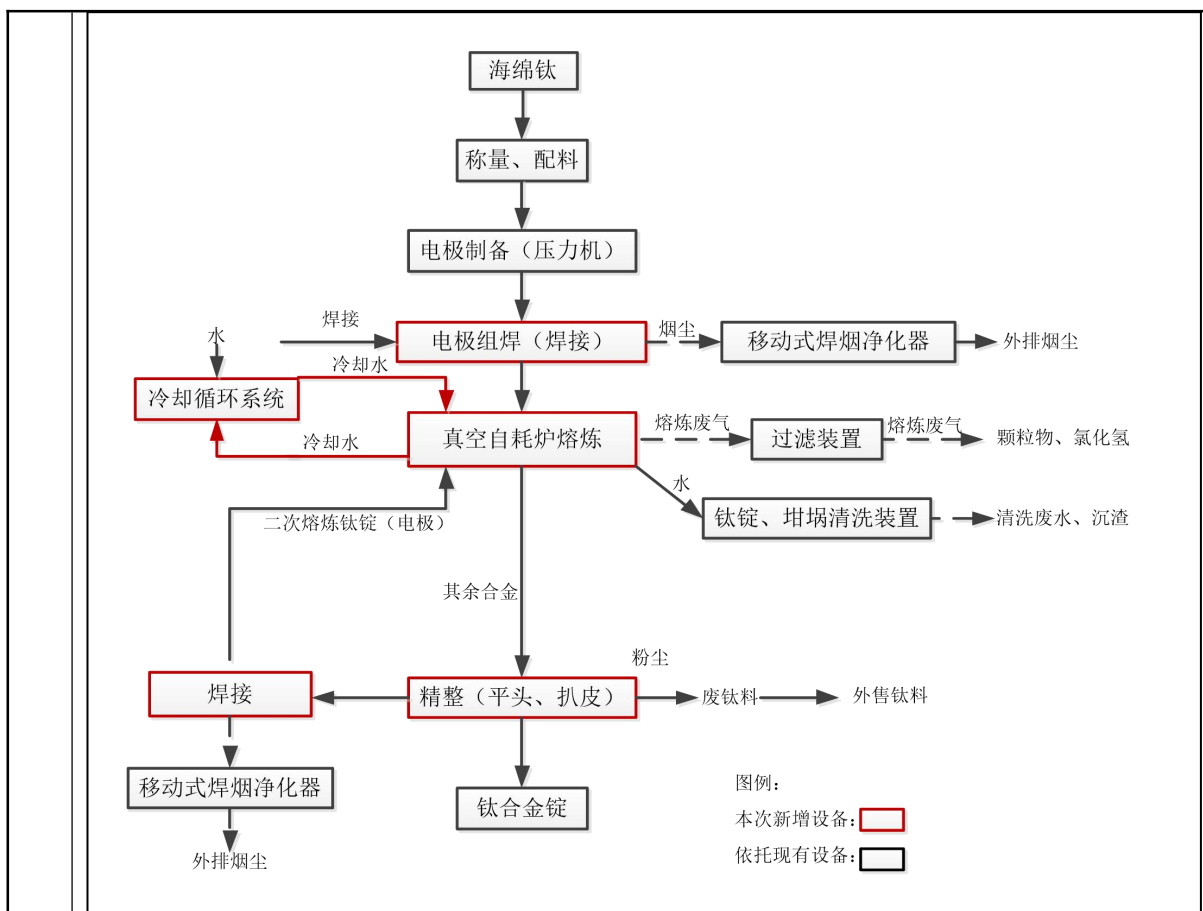
图 2-4 项目运营期钛锭生产工艺流程示意图
