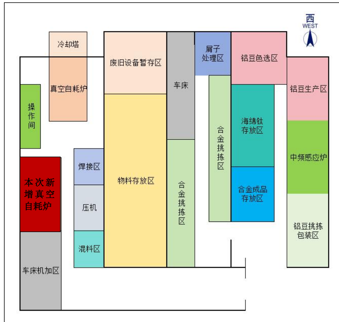
附图3 建设项目平面布局图
