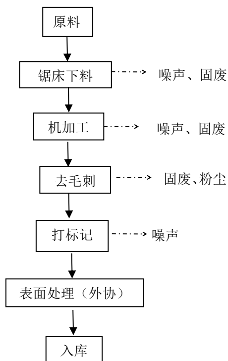
图 2-3 石油钻采专用设备的金属零部件加工工艺流程及产污环节图
