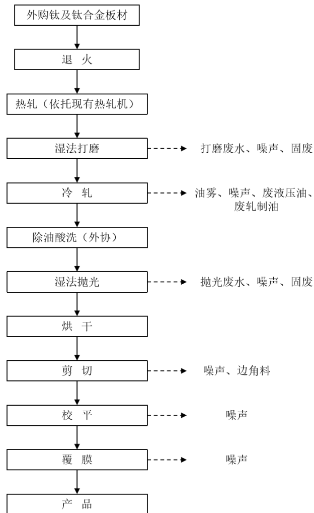
图 2-2 本项目运营期生产工艺流程及产排污环节示意图
