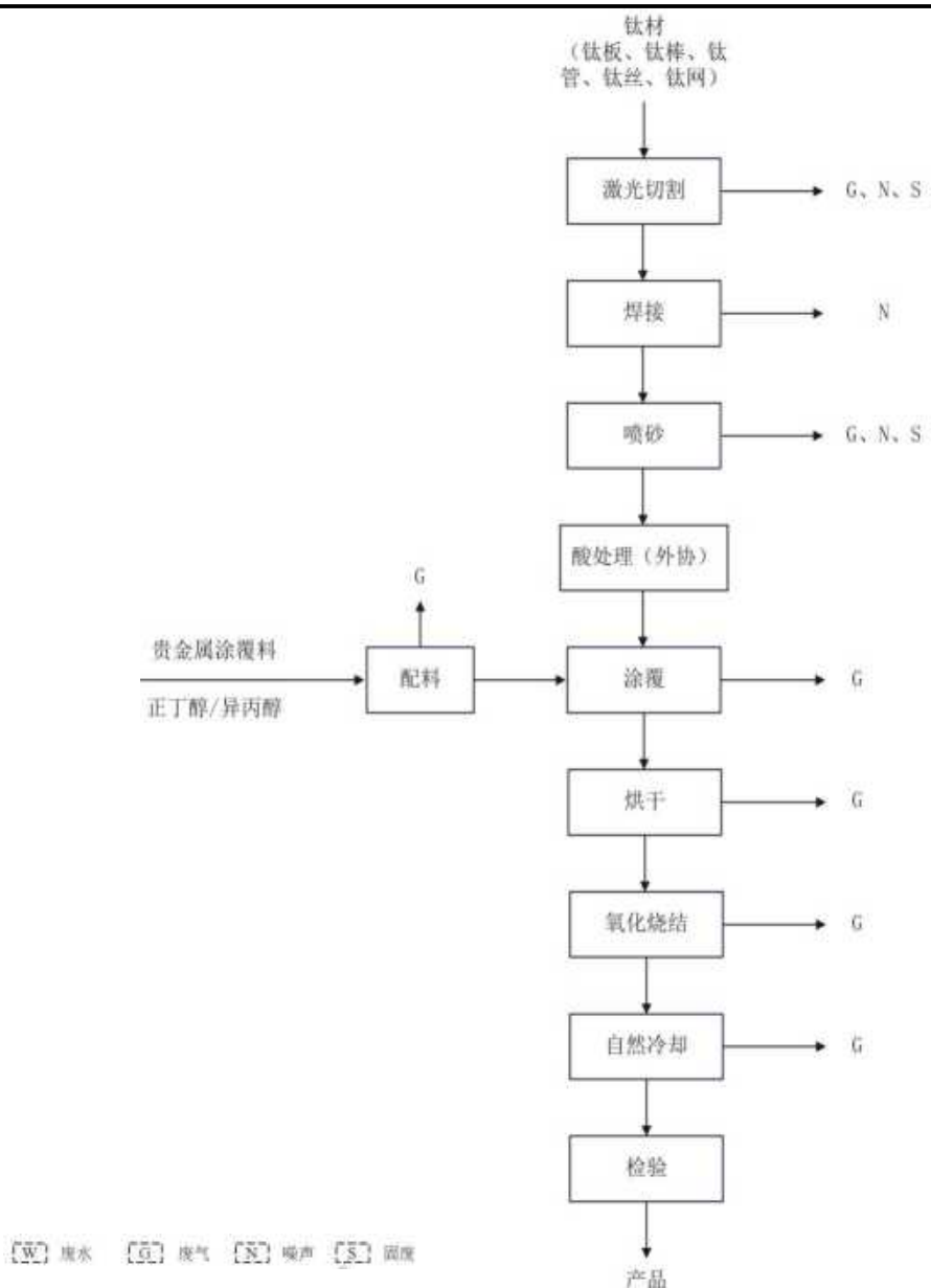
图 2-2 生产工艺流程及产污环节图
