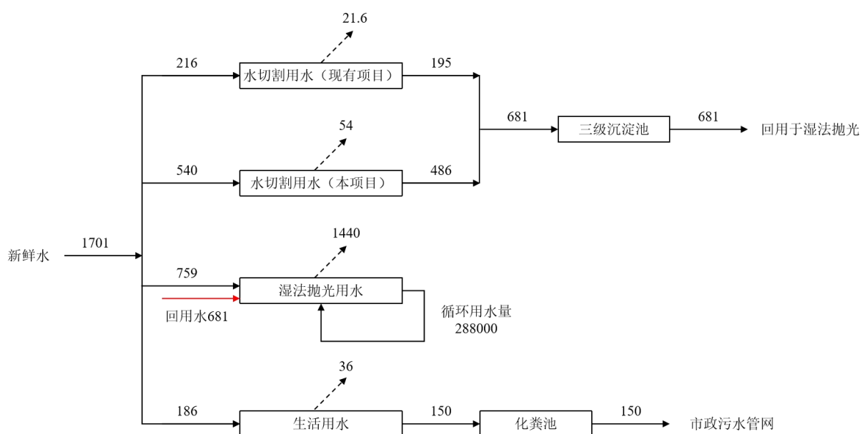
图 2-1 扩建项目建成后全厂水平衡图 单位：m³/a
