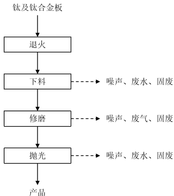
图 2-2 扩建项目运营期生产工艺流程及产排污环节示意图
