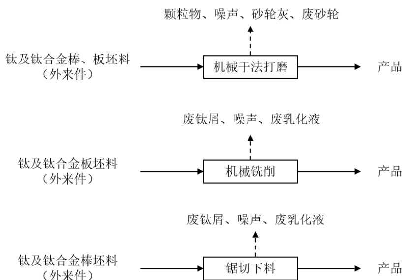
图 2-1 本项目生产工艺流程及产排污环节示意图
