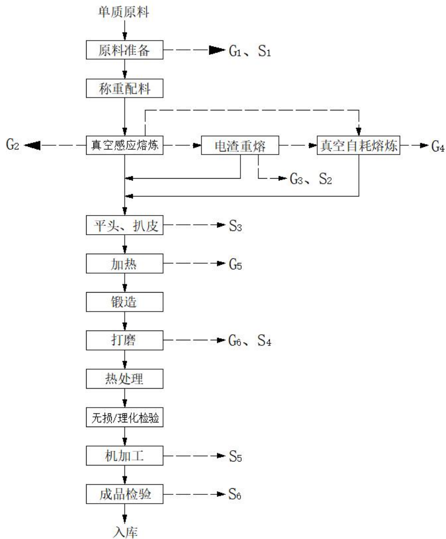
图 2-2 生产工艺流程及产污环节图
