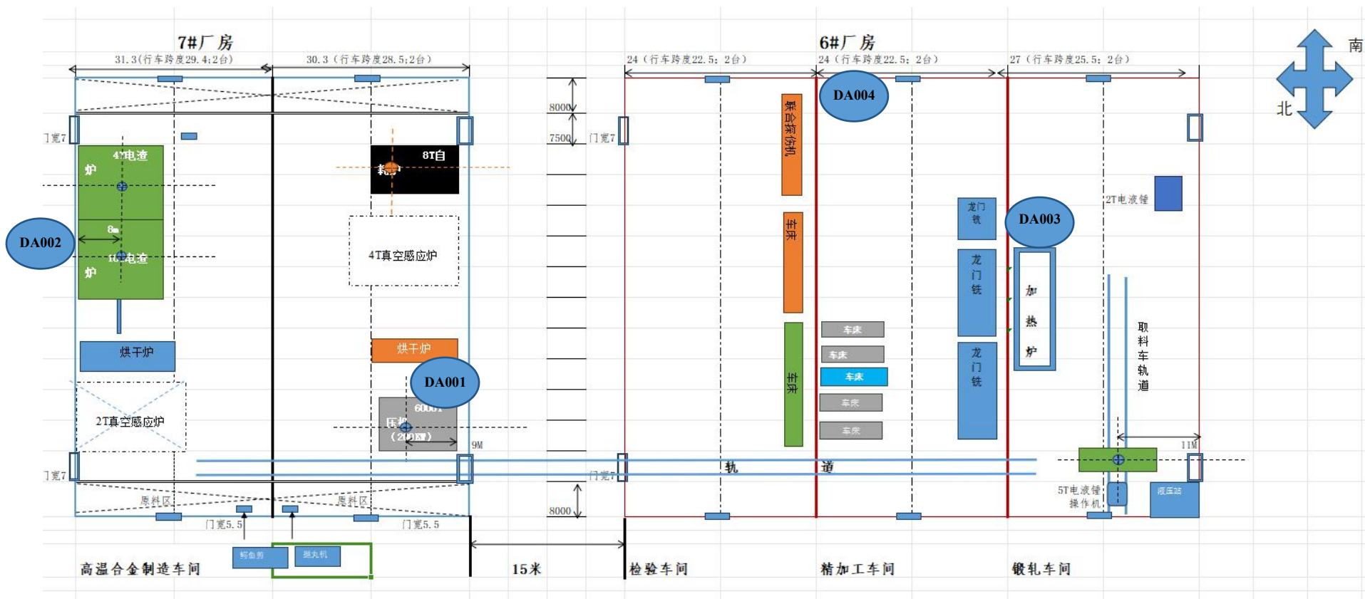
附图 4 建设项目厂区平面布置图
