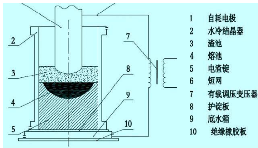
图1 电渣重熔原理图
