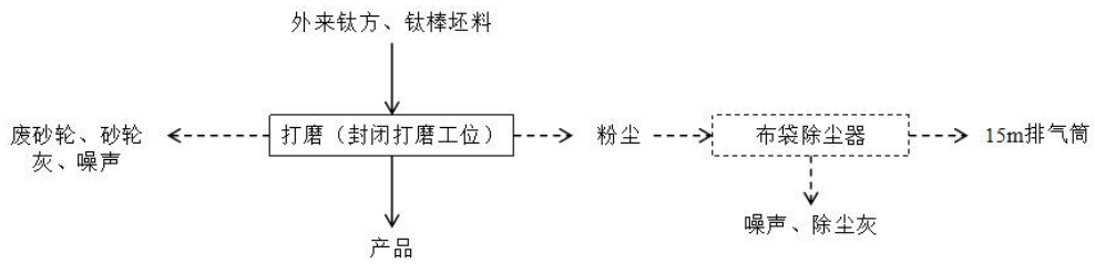
图 2-1 本项目生产工艺流程及产排污环节示意图
