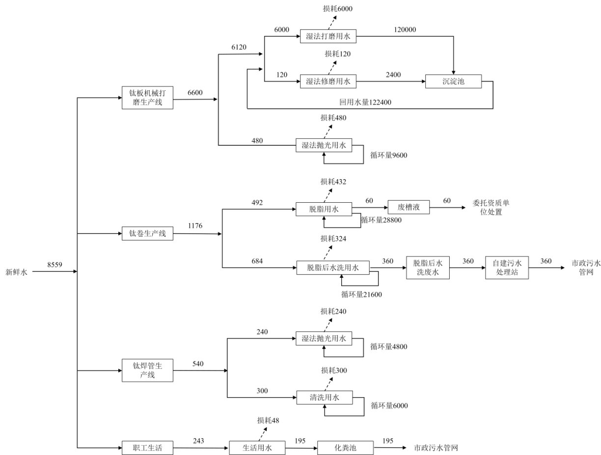
图 2-1 水平衡图 单位: m 3 /a
