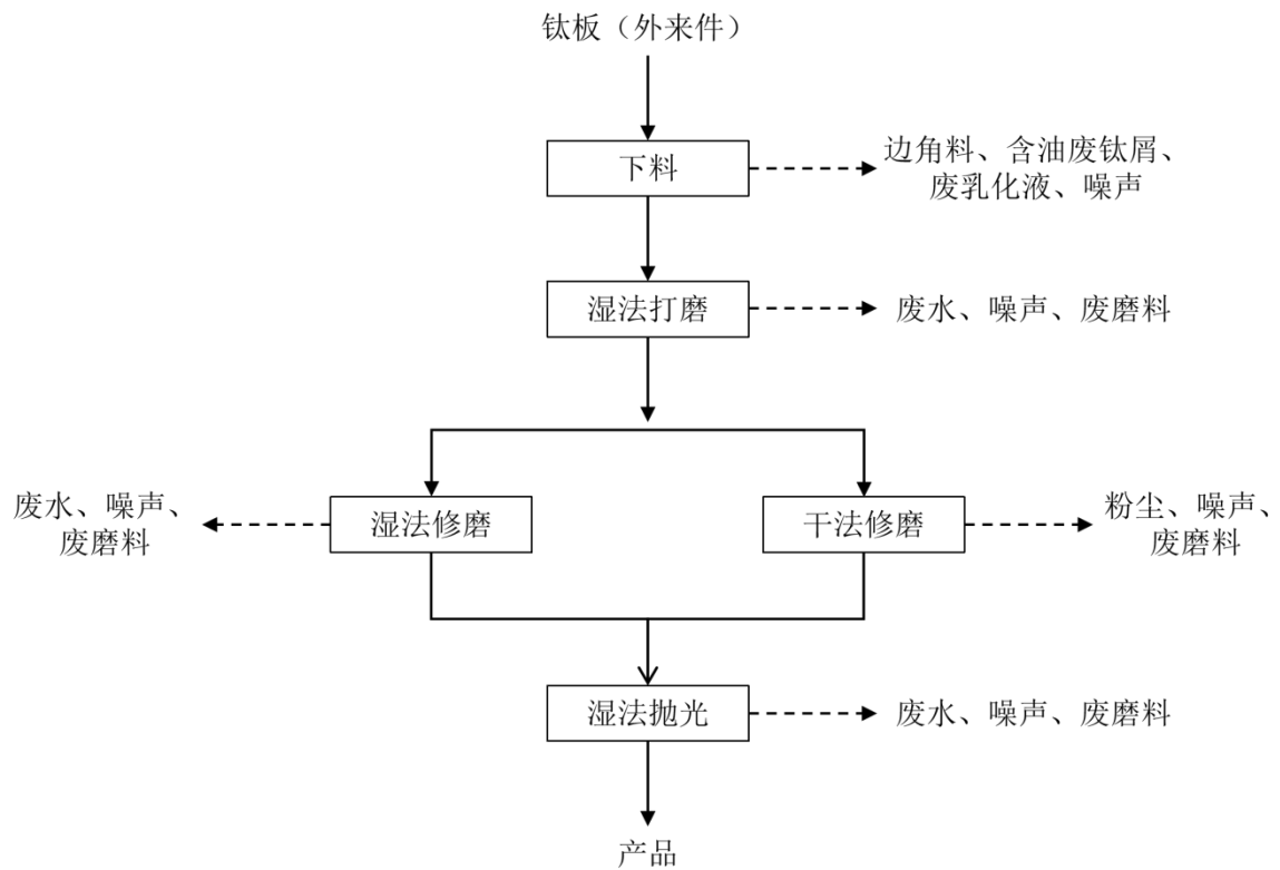
图 2-2 钛板机械打磨生产线工艺流程及产排污环节示意图
