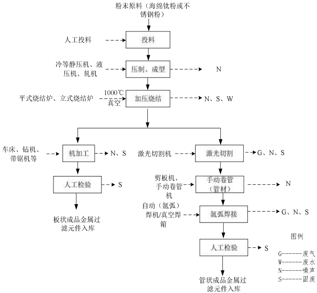
图 2-3 本项目生产工艺流程与产污环节图
