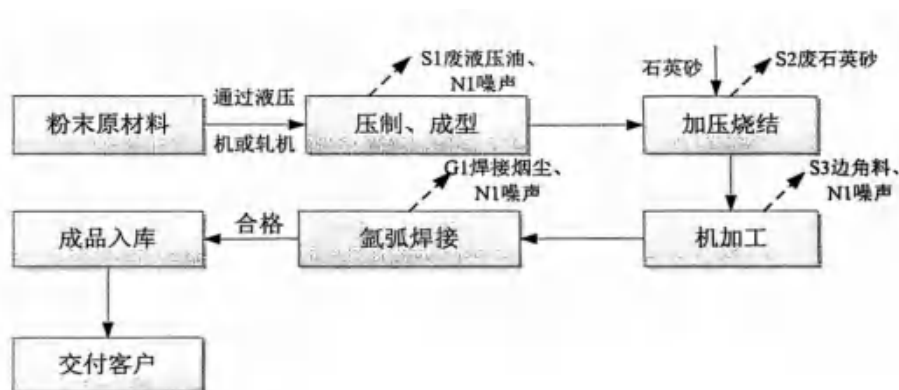
图 2-4 现有项目运营期主要生产工艺流程
