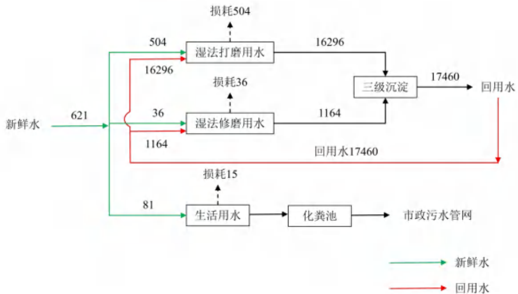
图 2-1 水平衡图 单位：m 3 /a
