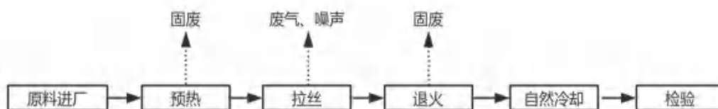
图 2-3 本项目热拉生产工艺流程图
