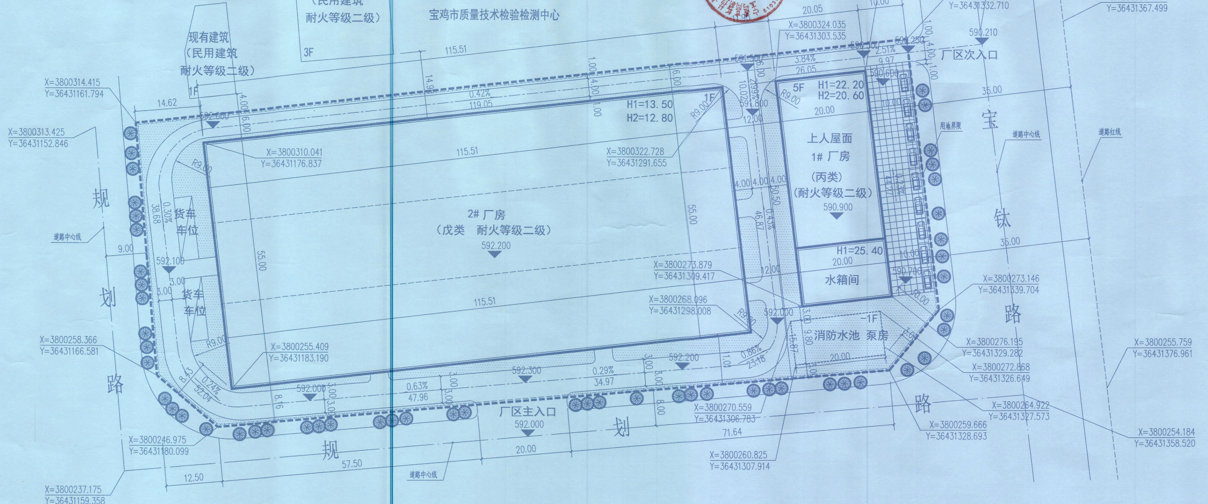
总平面图 1:500
