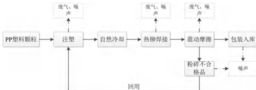
图 2-4 运营期工艺流程及产污环节图
