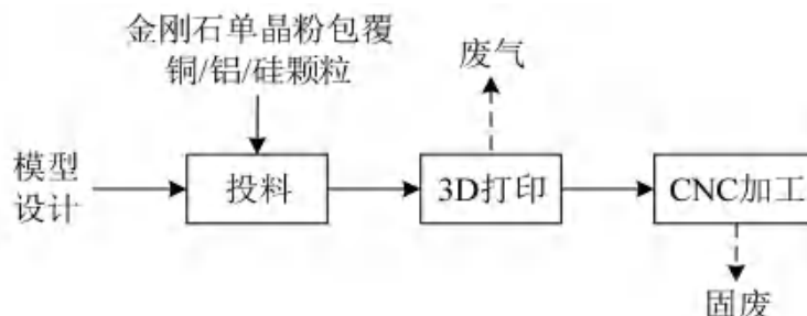
图 2-3 3D 打印工艺流程及产污环节示意图
