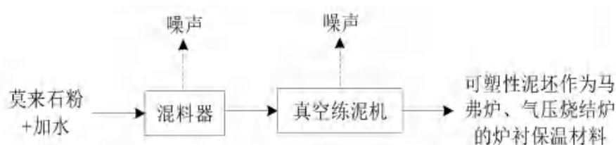
图 2-5 真空制泥工艺流程图
