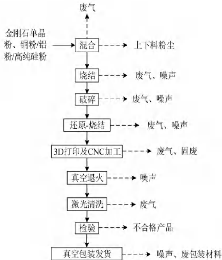
图 2-2 复杂形状的金刚石铜/铝/硅复合材料产品生产工艺流程图
