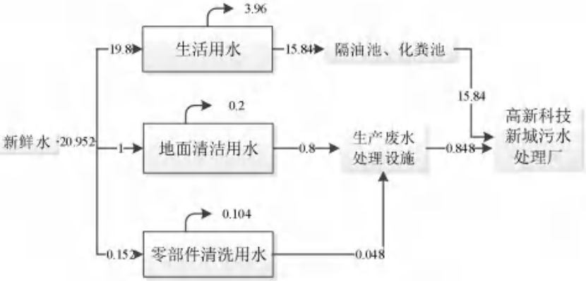
图 2-1 本项目水平衡图（m 3 /d）
