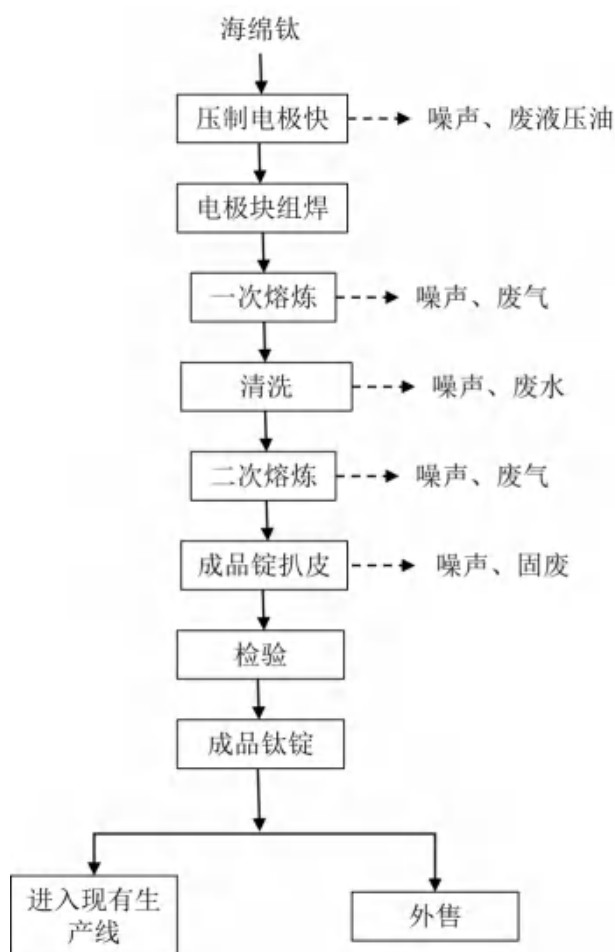
图 2-2 熔炼车间工艺流程和产排污环节示意图
