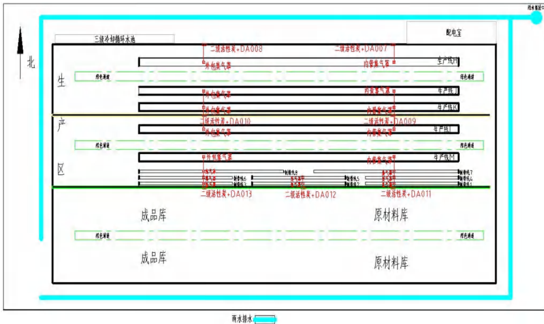
附图3 建设项目平面布置图（比例尺 1:800）
