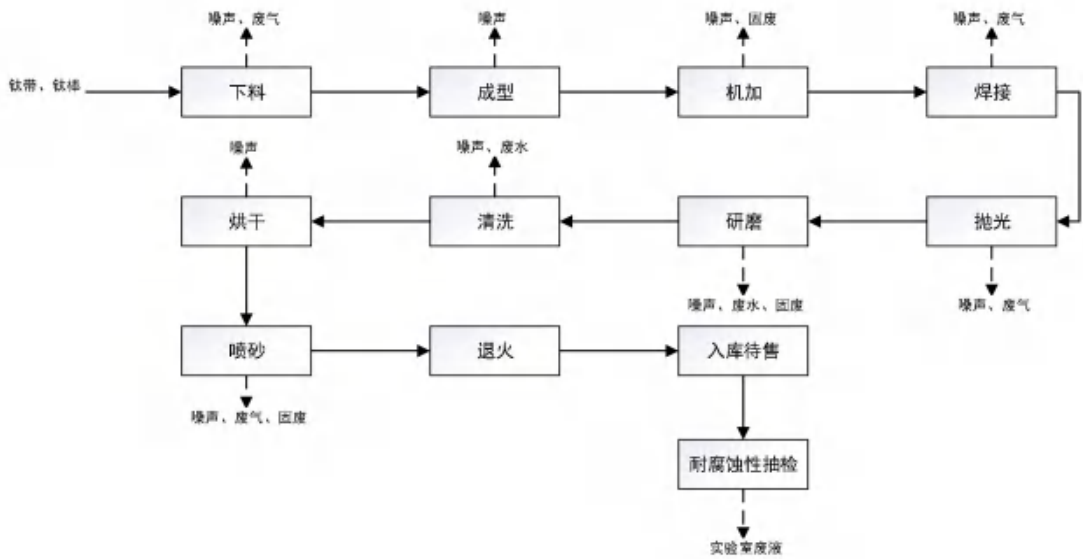
图 2-3 项目生产工艺流程及产污环节图
