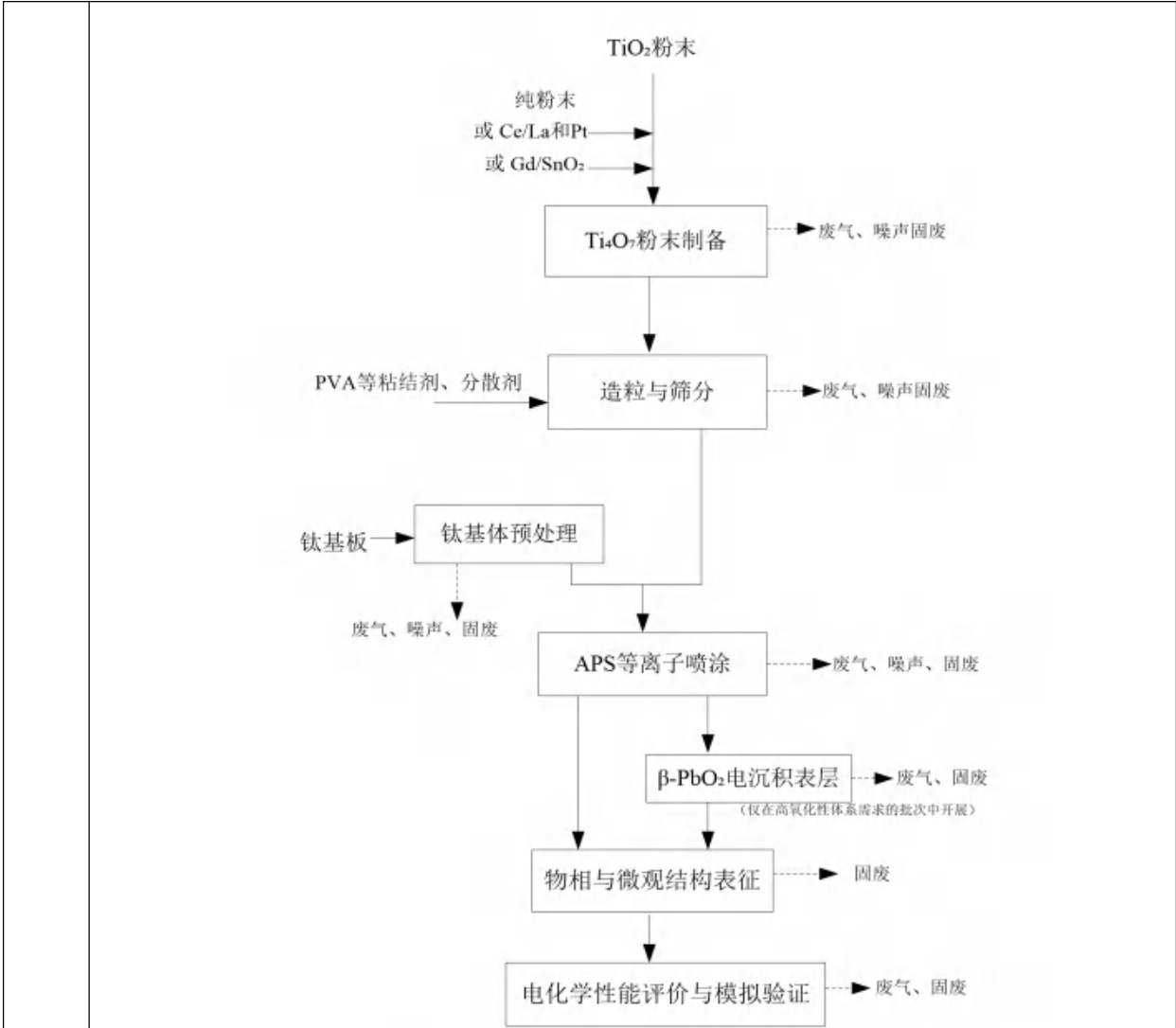
图2-5 \text{Ti}_4\text{O}_7 新型电极制备及性能评价流程图
