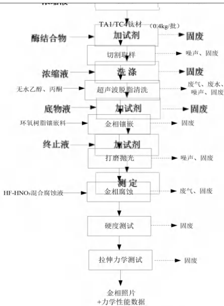
图2-3 钛材金相与力学性能检测流程图
