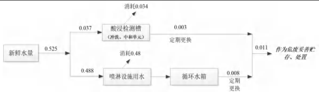
图 2-1 本项目水平衡图 (m³/d)
