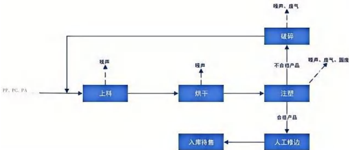
图 2-5 注塑线工艺流程及产污位置
