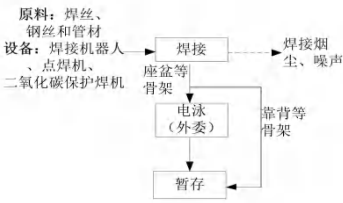
图 2-3 座椅骨架生产工艺流程及产污位置
