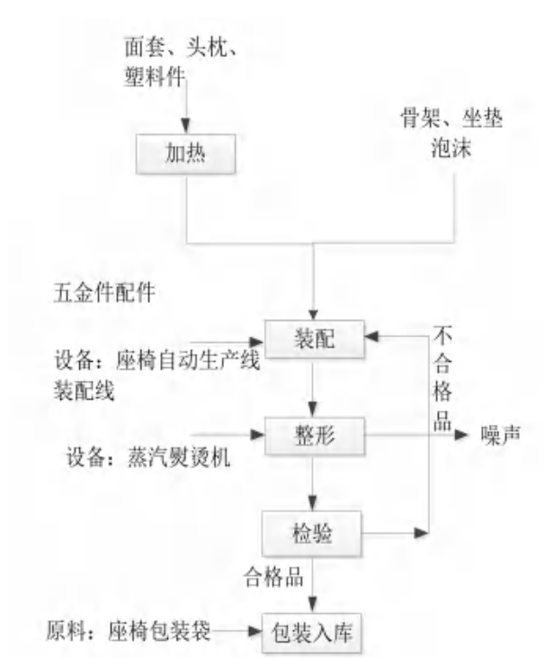
图 2-4 汽车座椅总装工艺流程及产污位置
