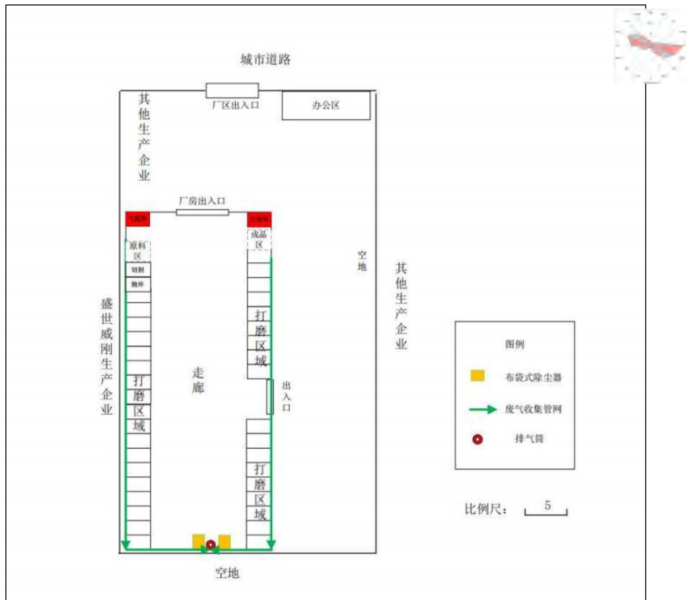
附图2 厂区平面布置图及四邻关系图
