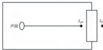
图 4-1 室内声源由室内向室外传播示意图
