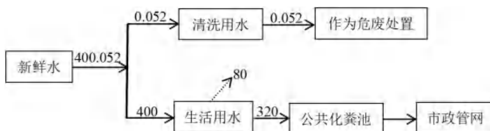
图 2-1 水平衡图 单位 m 3 /a
