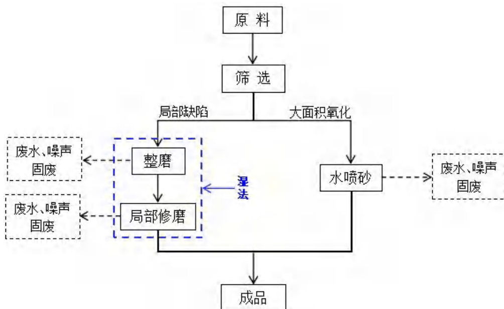
图 2-2 生产工艺流程及产污环节示意图
