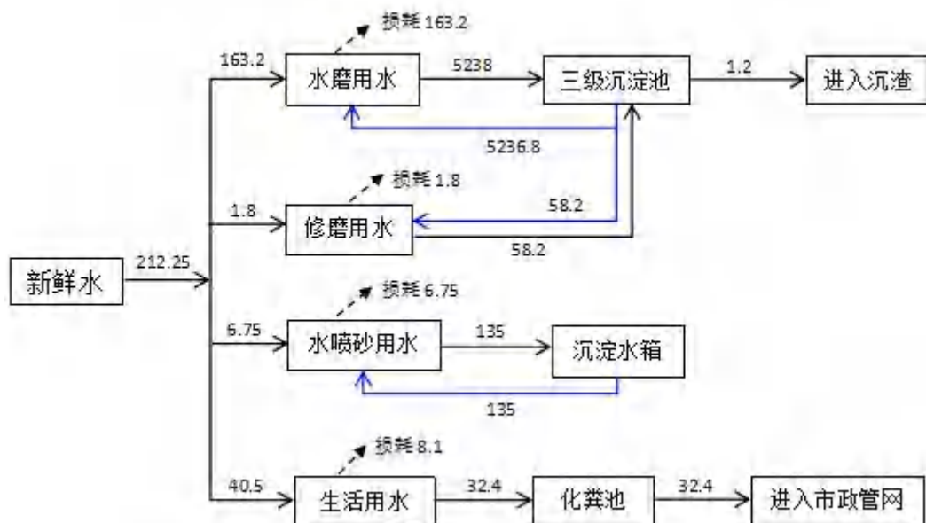
图 2-1 水平衡图 单位: \text{m}^3/\text{a}
