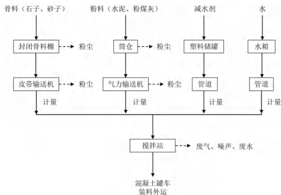
图 2-2 本项目生产工艺流程及产排污环节示意图
