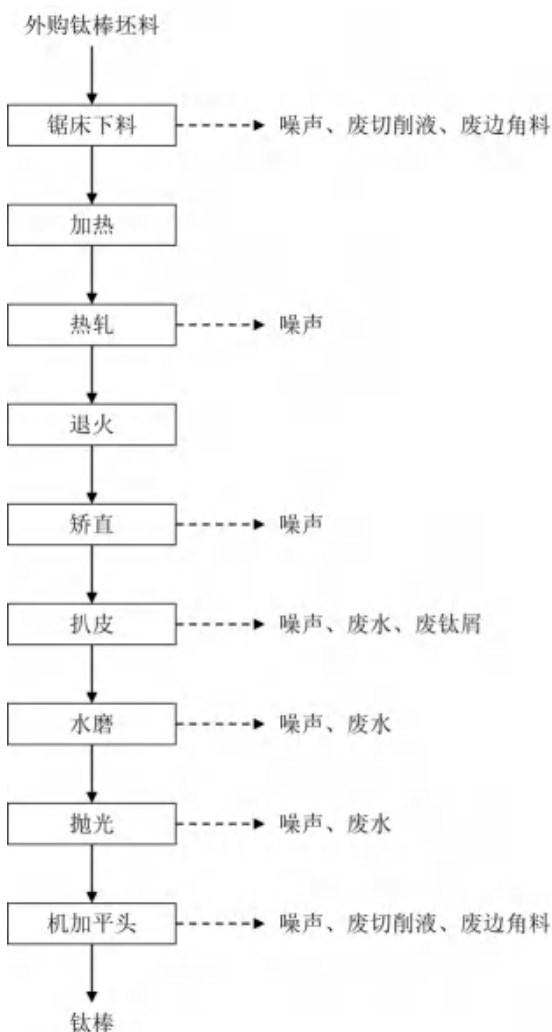
图 2-2 本项目运营期工艺流程及产排污环节示意图
