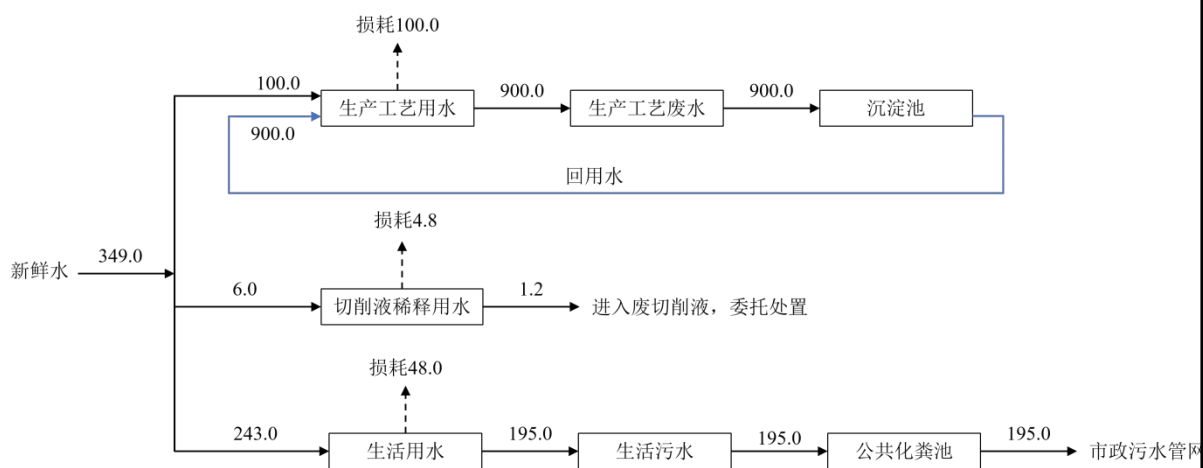
图 2-1 水平衡图 单位：m 3 /a
