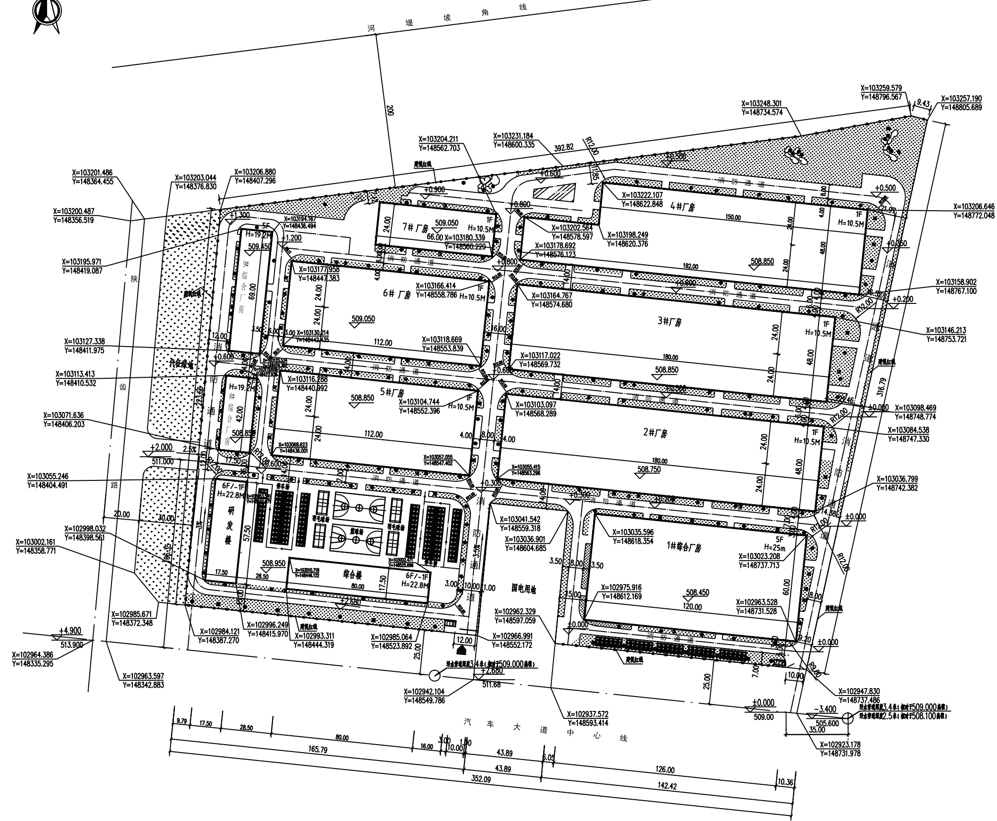
总平面图 1:1000
