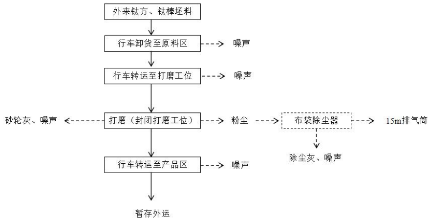
图 2-1 本项目生产工艺流程及产排污环节示意图
