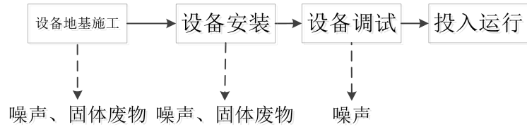
图 2-2 项目施工期工艺流程及产污环节图
