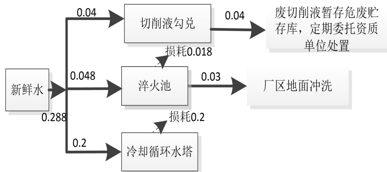
图 2-1 项目水平衡图 (d/a)
